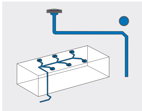
Pluvia takavvanningssystem med undertrykk
