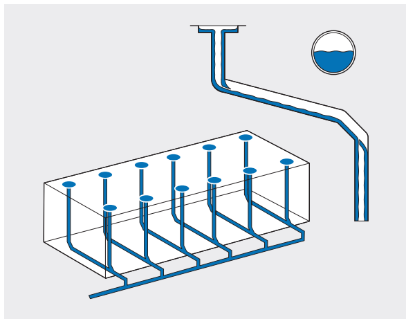
Konvensjonelt takavvanningssystem
